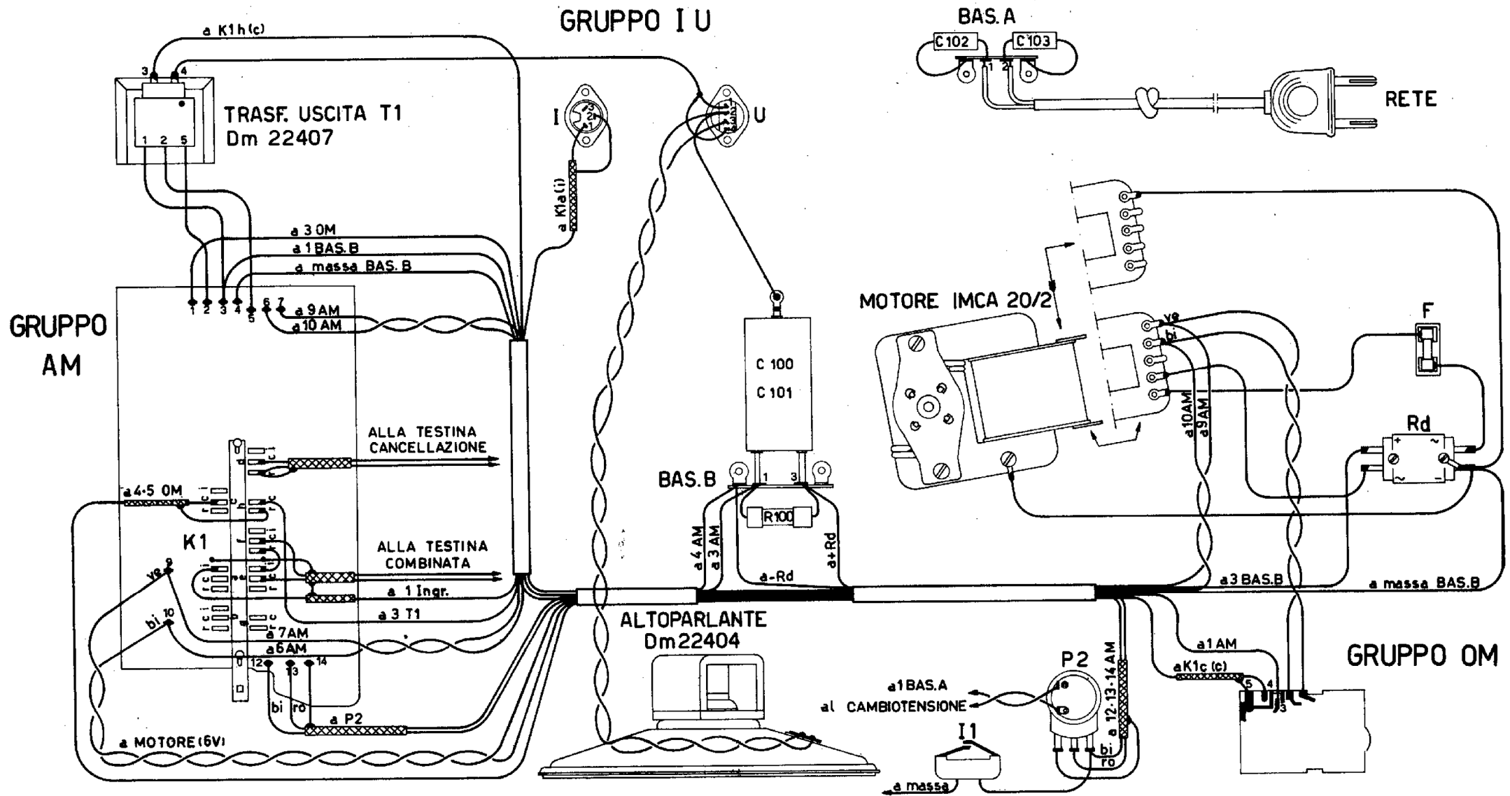
Fig. 3 - Cablaggio Renas C2.
